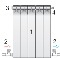
Нижнее подключение
